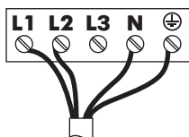
Võrguvoolu ühendus 2-faasiline
