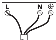
Võrguvoolu ühendus 1-faasiline
