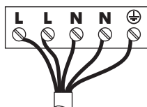
NL Võrguvoolu ühendus 2-faasiline
